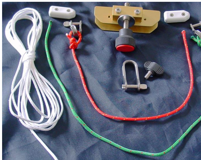
Montage-Set für Motor- und Fahrhebel-Halter inkl. Steuerseil-Verbindung, Schäkel, Süllrand-Halter für Fahrhebel-Plattform inkl. Schraube, Set 63,20 € inkl. MwSt. zzgl. Versandkosten
